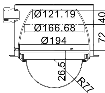
內部尺寸圖
