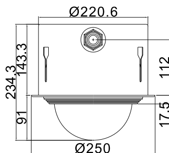
外部尺寸圖
