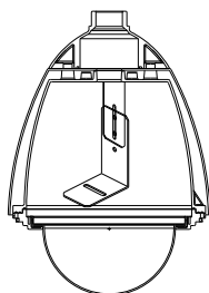
固定式攝影機安裝方式
