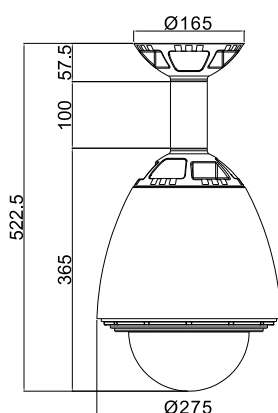
外部尺寸圖
