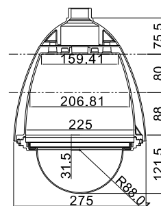
內部尺寸圖
